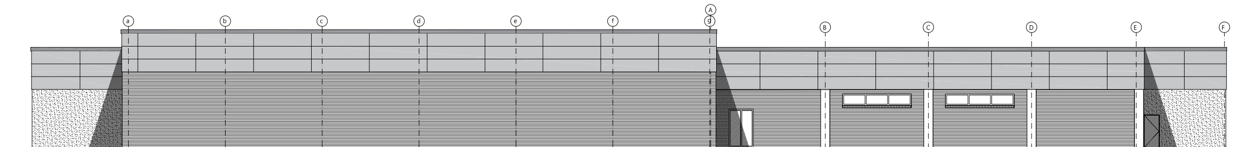
Nordansicht
