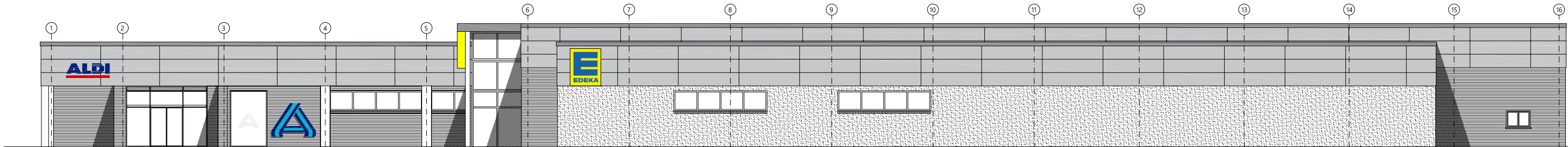
Ostansicht
